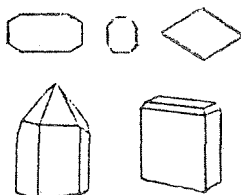
ORTHORHOMBIC
