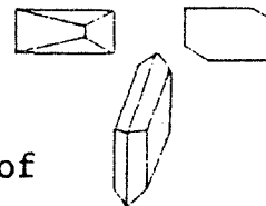
MONOCLINIC
